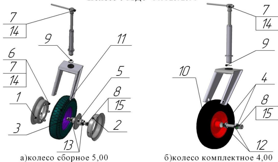
Рисунок 5. Колесо УМДУ-80/82.02.06
